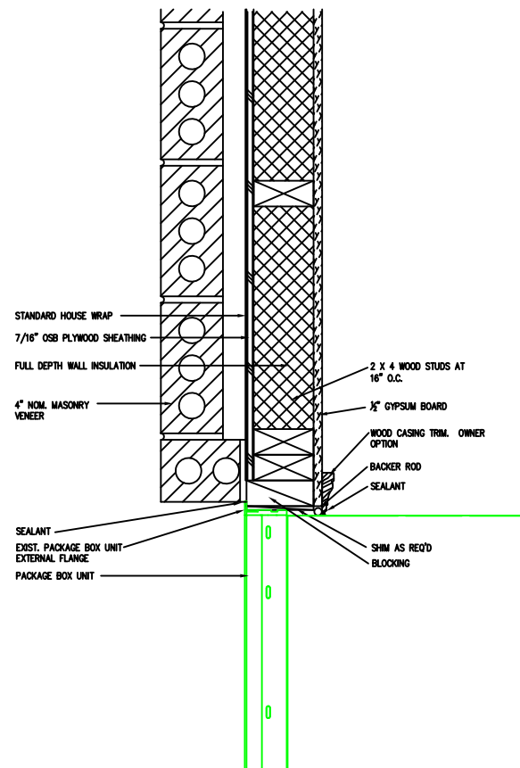
JAMB DETAIL
